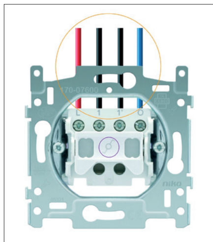
Obr. 8. Umístění připojovacích svorek na jedné straně
